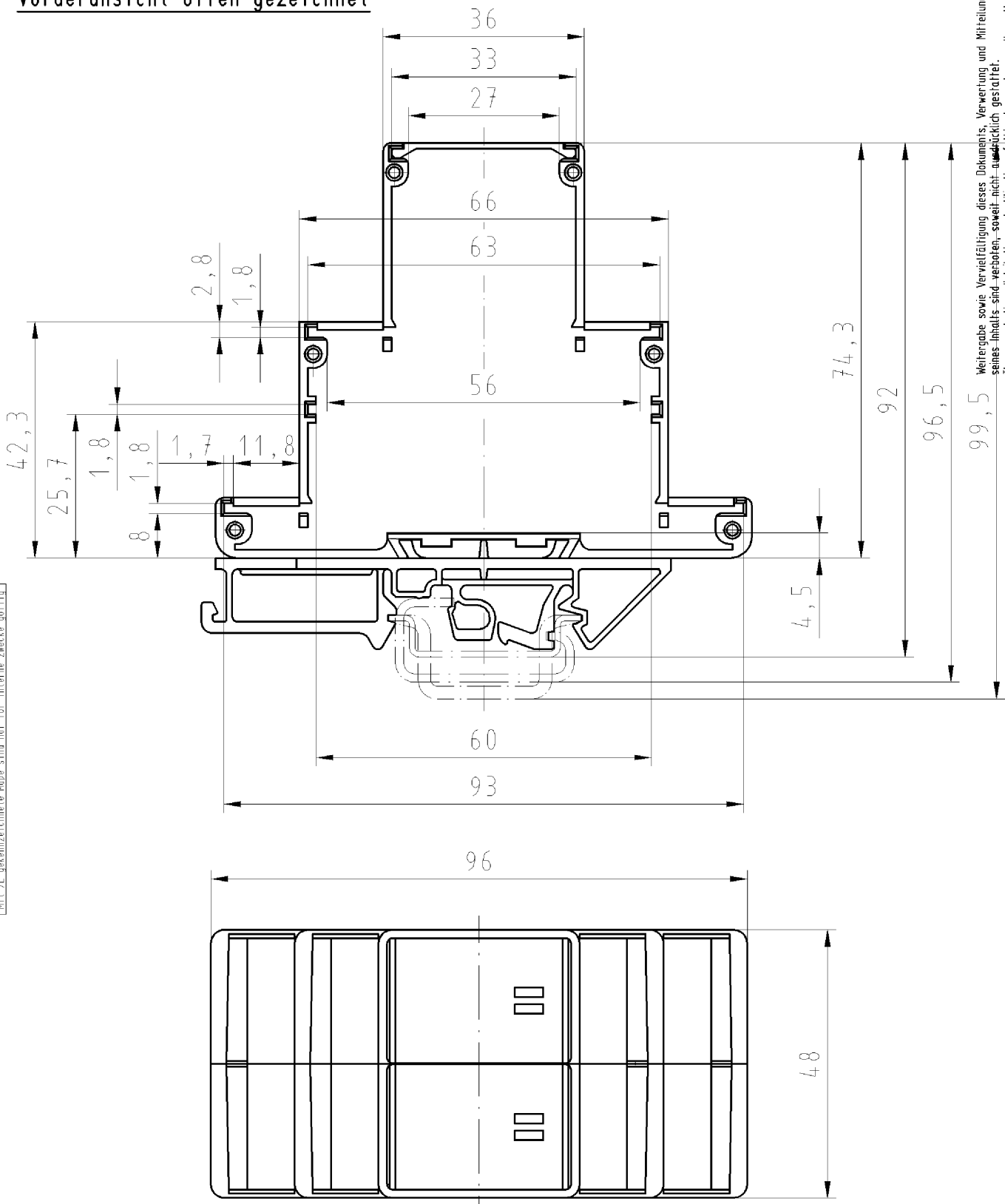
Abmaße für Platine 93/63x45 Dimensions for PCB 93/63x45
