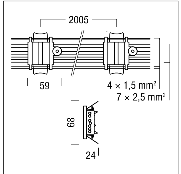
ZS_TRS_M_Verdrahtung_11pol_2000.wmf
