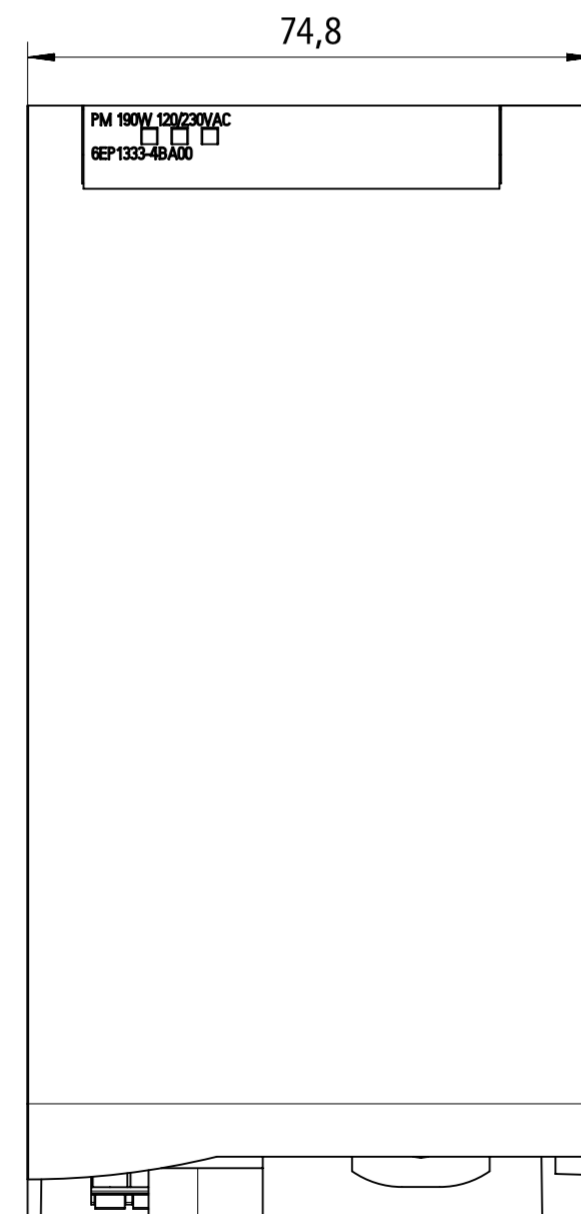
Vorne / Front
