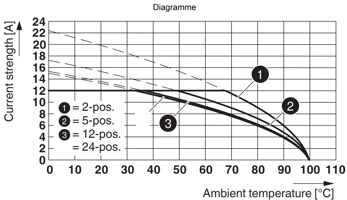
Type : MVSTB(R/W) 2,5/...-ST avec MDSTBVA 2,5/...-G-5,08
