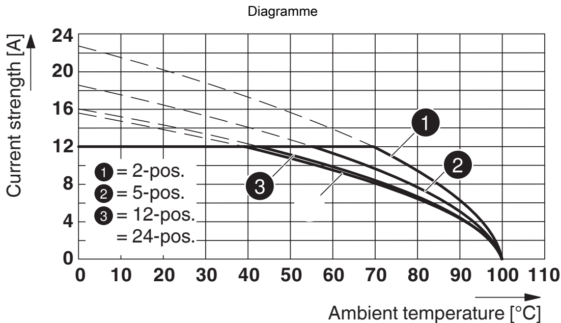
Type : MSTBU 2,5/...-STD-5,08 avec MSTB 2,5/...-G-5,08
