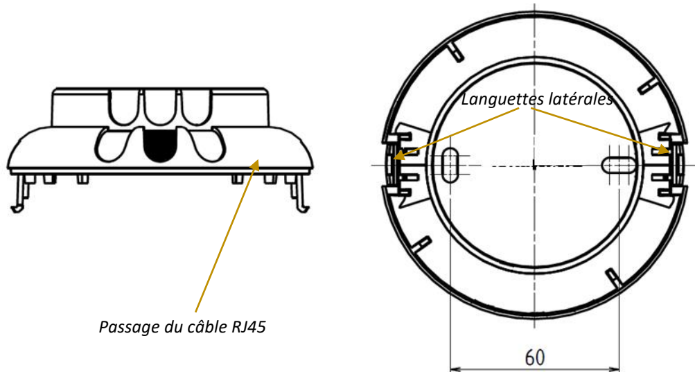
Fig. VI : Fixation murale du GZ-CAPT1
