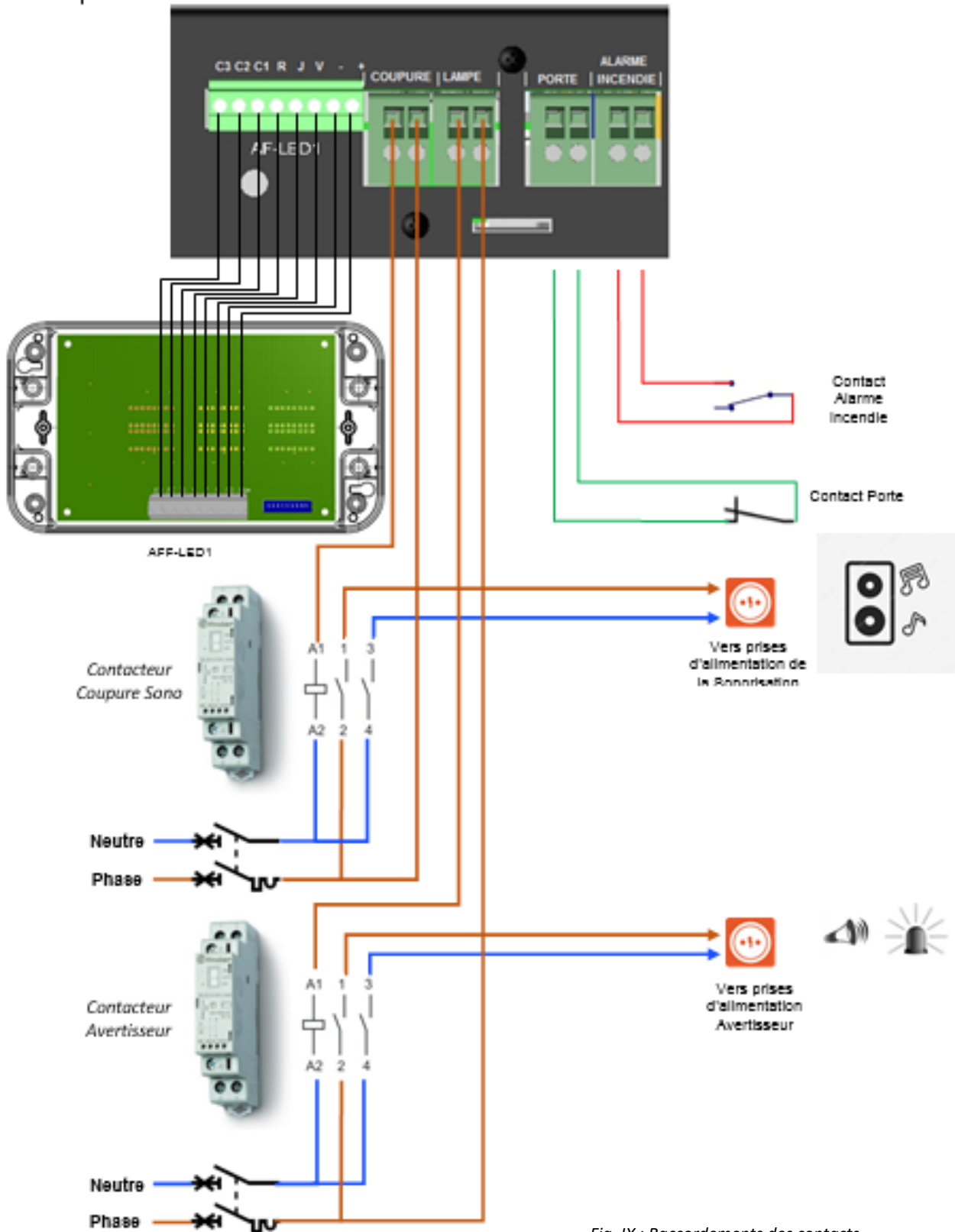
Fig. IX : Raccordements des contacts
