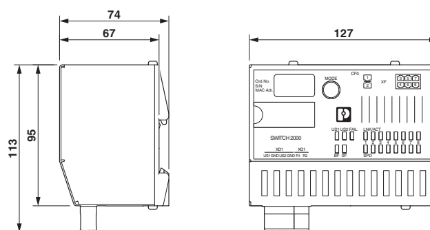
Dessin coté
