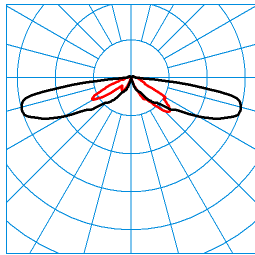
8841 AB14L/700-730 2G2 ETDD (CLOENDWERT) TX369288 ■ C0 - C180 ■ C90 - C270 DIN 5040: A10 UTE: 0,94 J + 0,06 T CEN Flux Code: 10 35 79 94 100 9 31 58 6
