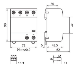
Dimensions DSH TNS 255 FM
