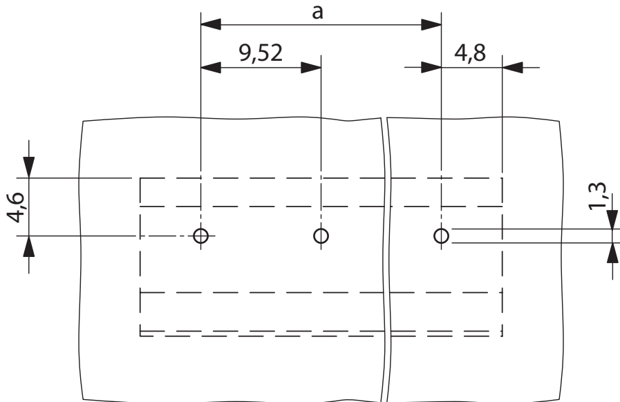
Dessin coté
