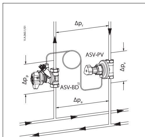
Fig. 1 Réglage de la vanne ASV-PV = \Delta p_{colonne} (Vanne associée à l'extérieur du circuit de contrôle)
