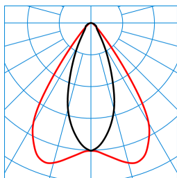
E-Line PRO 78IP50 MironaF HR 270-840 ETDD L225 01 ESG 01 (LEO3) TX720718 ■ C0 - C180 ■ C90 - C270
