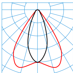
E-Line PRO 78IP50 MironaF HR 270-840 ETDD L225 01 ESG Blank (LEO1) TX720719 ■ C0 - C180 ■ C90 - C270
