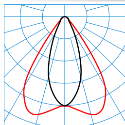
E-Line PRO 78IP50 MironaF HR 270-840 ETDD L225 01 ESG 01 (LEO1) TX720716
