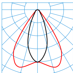
E-Line PRO 78IP50 MironaF HR 270-840 ETDD L225 01 ESG Blank (LEO2) TX720720 ■ C0 - C180 ■ C90 - C270
