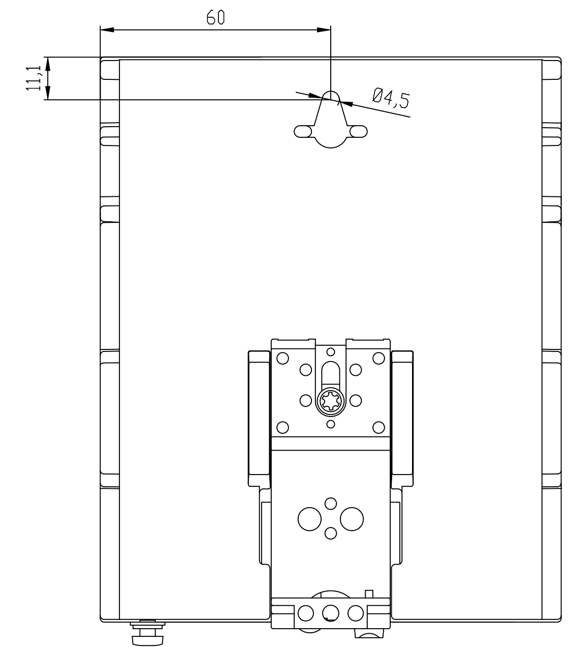
Hinten / Back
