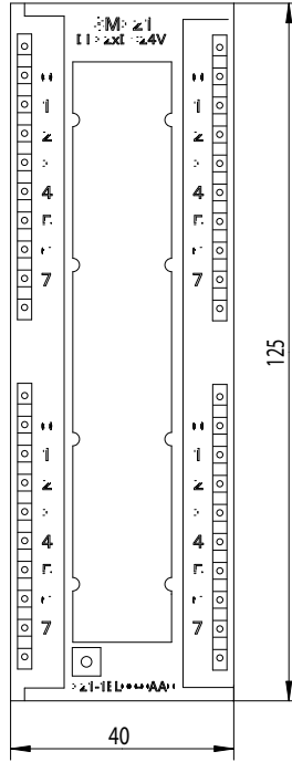
Vorne / Front
