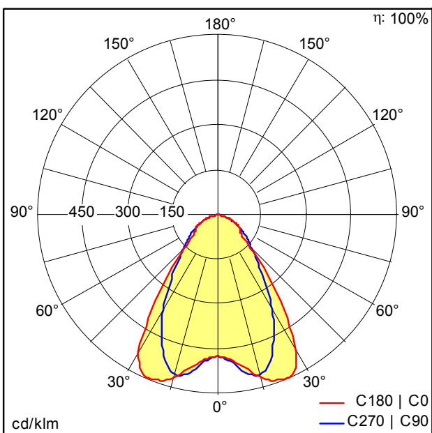
D44421AA_TEC_LED3700-865_L1000_WB_LDE_WH_IP.ltd
