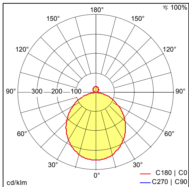
D38116AA_ONDA2_A_AV_D870_LED6400-840.Idt
