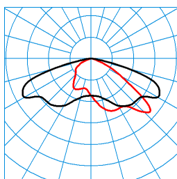
Jovie 70-AB7L-LR/10000-740 8G1 ET (CLO initial value) TX301665 ■ C0 - C180 ■ C90 - C270 DIN 5040: A30 UTE: 1,00 G CEN Flux Code: 34 71 96 100 100
