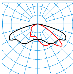
Jovie 70-AB7L-LR/10000-740 8G1 ET TX068601 ■ C0 - C180 ■ C90 - C270 DIN 5040: A30 UTE: 1,00 G CEN Flux Code: 34 71 96 100 100
