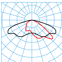
Jovie 70-AB7L-LR/10000-740 8G1 ET (CLO end value) TX300391 ■ C0 - C180 ■ C90 - C270 DIN 5040: A30 UTE: 1,00 G CEN Flux Code: 34 71 96 100 100
