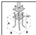
S.2849 Embase de fixation à sceller pour POTEAU S.2801, S.2813, S.2843, S.2845 à sceller en acier zincu  avec visserie M16, C= 200mm, D=200mm E= 80mm, h=460mm, h1=90mm. Il est conseillé de sceller cette embase dans le b ton selon les dimensions ci-dessous **: A = 0.7 m B = 0.7 m **Les dimensions du bloc de b ton peuvent varier en fonction de la nature du terrain, selon les indications de la norme UNI EN 40.
