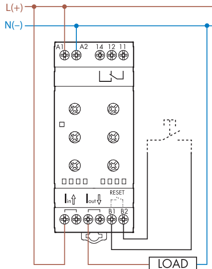
Type 70.51 et 70.51 NFC
