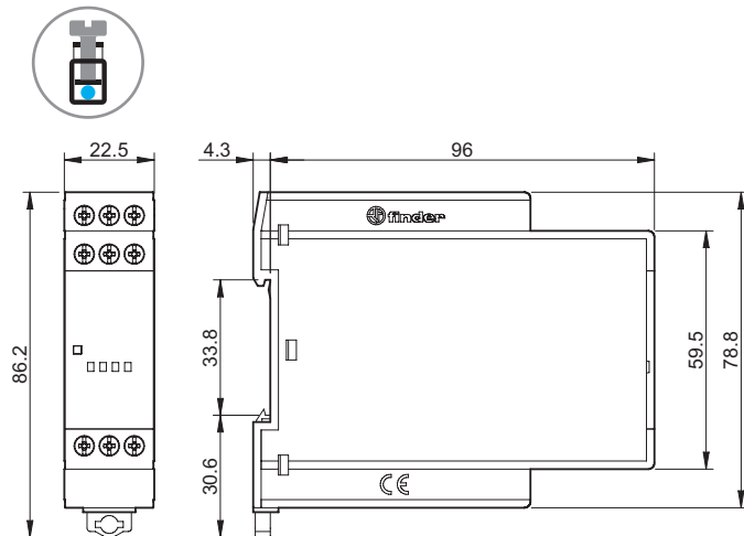
Type 70.62 Bornes à cage
