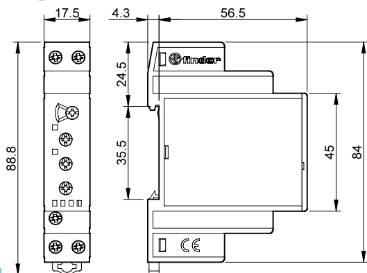
Type 70.41 Bornes à cage
