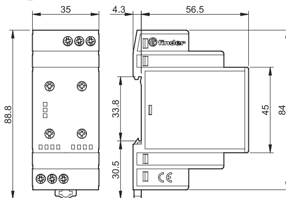
Type 70.42 Bornes à cage
