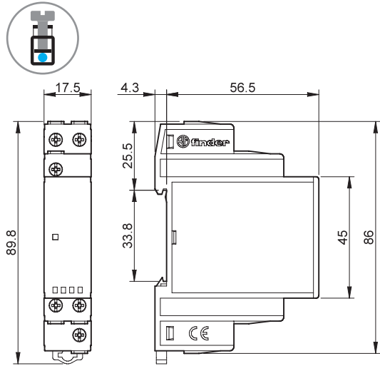
Type 70.62 Bornes à cage
