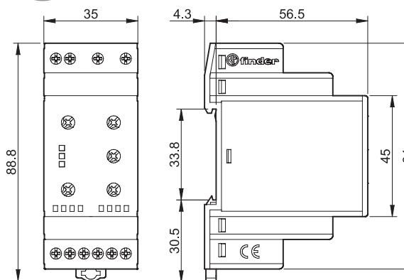
Type 70.51.0.240.N032 Bornes à cage
