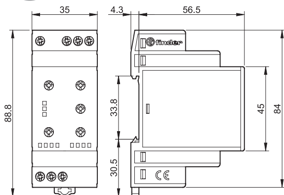
Type 70.51.0.240.2032 Bornes à cage
