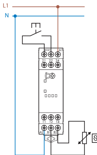
Type 70.51 et 70.51 NFC
