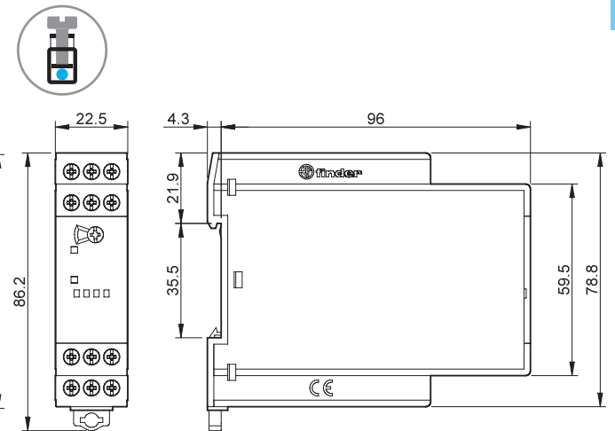
Type 70.92 Bornes à cage
