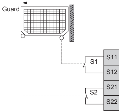
Garde / Schutzeinrichtung / Dispositivo / protector / Protezione / 防护
