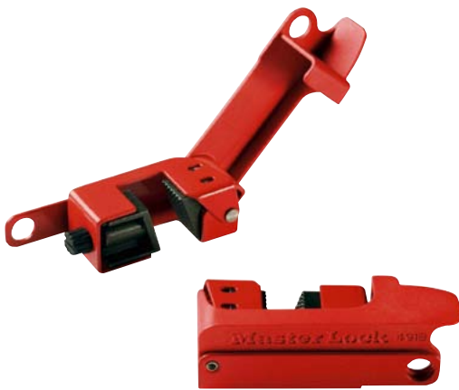
Pour disjoncteur à maneton simple et double standard.
