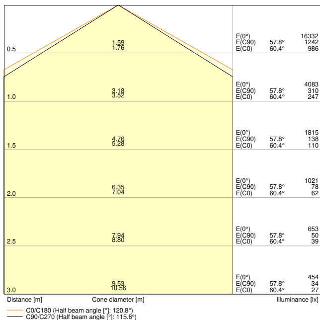
LB FLEX 1500 DALI P 73W 840 VW
