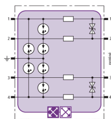
Schéma de principe du circuit BXT ML4 BD EX 24
