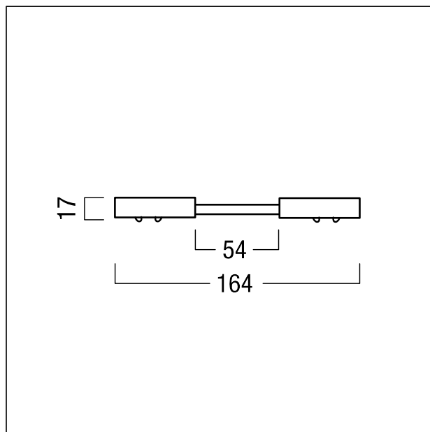
ZS_SU2_M_Leit_Bruecke.wmf
