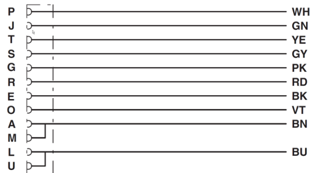
Kontaktbelegung der M16-Buchse
