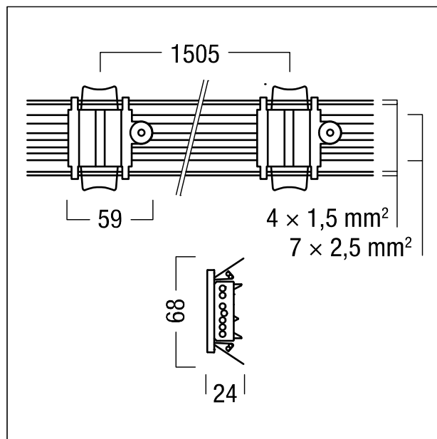
ZS_TRS_M_Verdrahtung_11pol_1500.wmf
