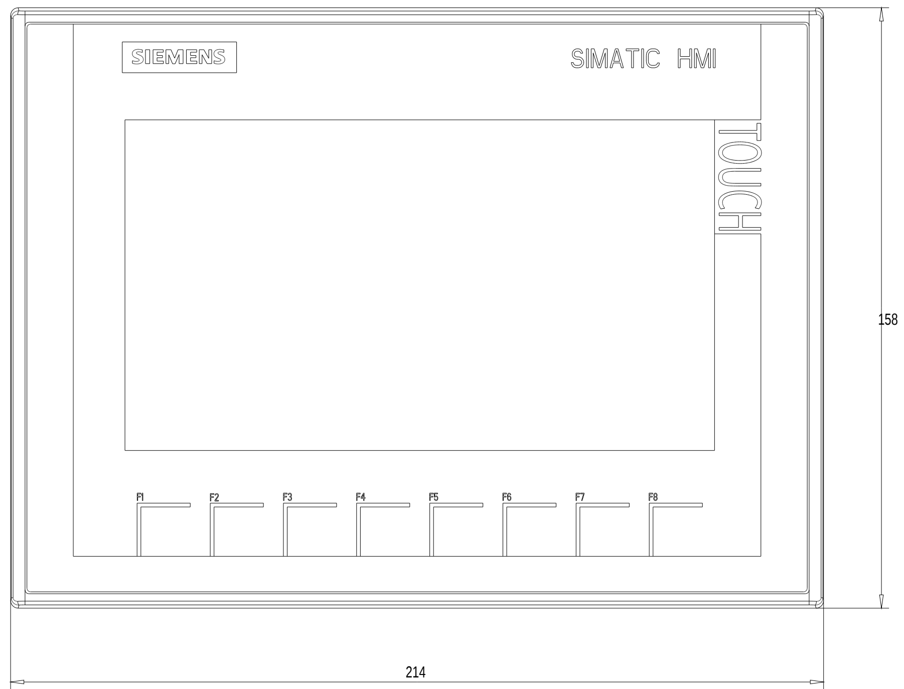
Vorne / Front
