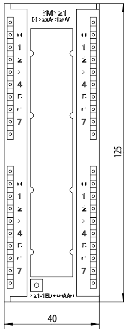
Vorne / Front
