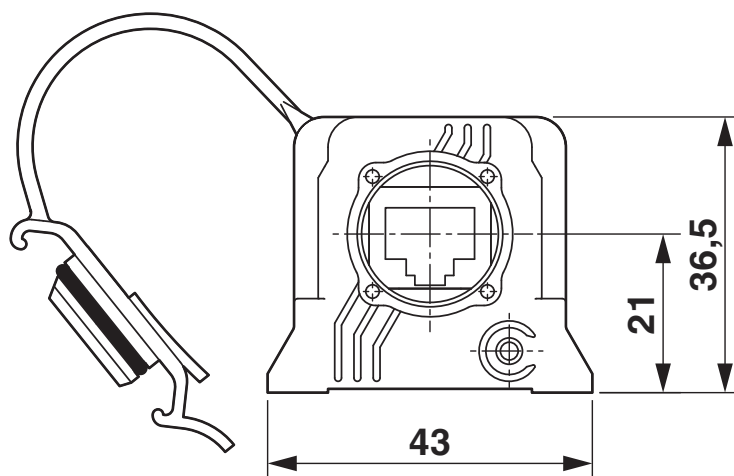
Dessin coté
