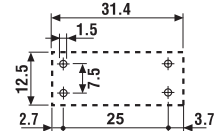
Vue côté cuivre
