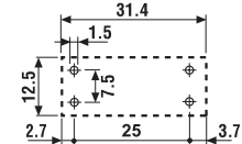
Vue côté cuivre
