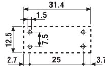
Vue côté cuivre
