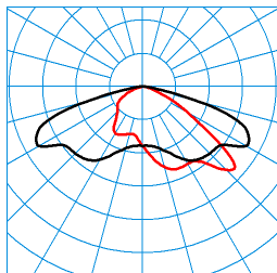
Jovie 70-AB7L-LRA/13500-740 12G1 ET (CLO end value) TX300426 ■ C0 - C180 ■ C90 - C270 DIN 5040: A30 UTE: 1,00 G CEN Flux Code: 34 72 96 100 100
