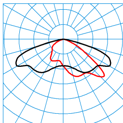
Jovie 70-AB7L-LRA/13500-740 12G1 ET (CLO initial value) TX301270 ■ C0 - C180 ■ C90 - C270 DIN 5040: A30 UTE: 1,00 G CEN Flux Code: 34 72 96 100 100
