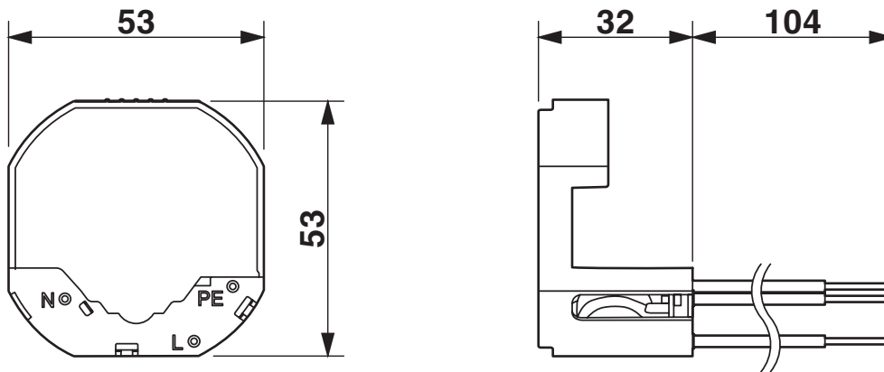
Dessin coté
