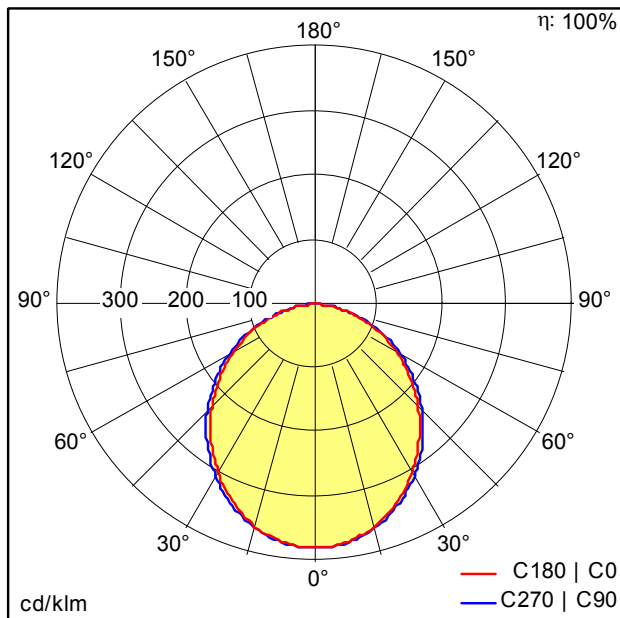
D33717AA_SLOT2_B_LED840_L1200_PM.Idt
