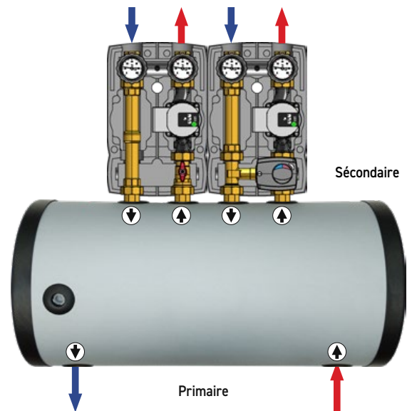
Schéma d'application: bouteille montage horizontal
