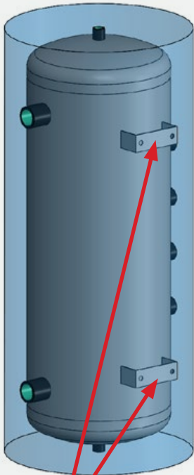
Supports de fixation murale fournis en standard.
