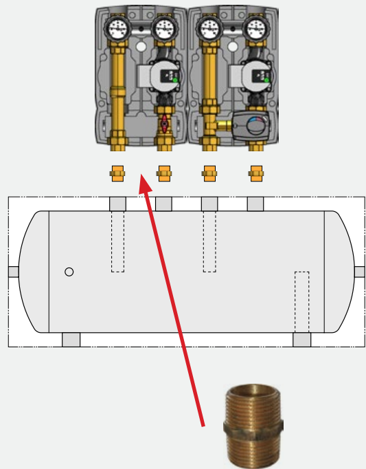
Pour le raccordement des modules, il est nécessaire d'utiliser des mamelon égal 1" (non inclus dans la fourniture standard).
