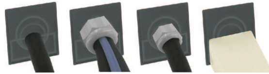
Embouts défonçables/Pre-punch hole plate Direct/direct input - Pour/for PG32 - Pour/for PG16 - Goulotte PVC/trunk 40x20 mm
