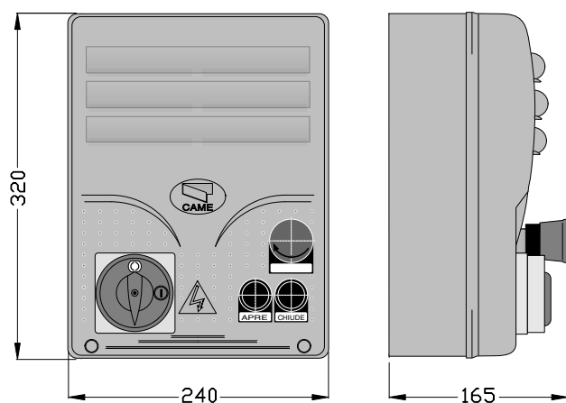
Encombremments boîtier ZT6C
