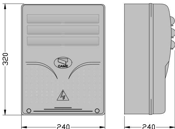
Encombremments boîtier ZT6
