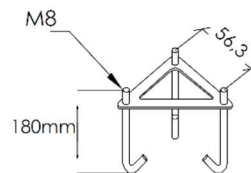
Art. 205ZZ Ancre pour béton Acier galvanisé
