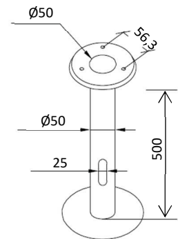
Art. 206ZZ Ancre pour sol meuble Acier galvanisé
