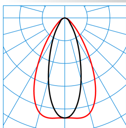
E-Line PRO 78IP50 MironaF T 270-840 ET L225 01 ESG 01 (LEO1) TX720030
