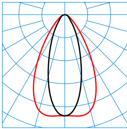
E-Line PRO 78IP50 MironaF T 270-840 ET L225 01 ESG 01 (LEO2) TX720035
