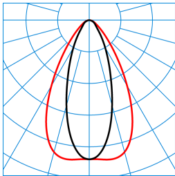
E-Line PRO 78IP50 MironaF T 270-840 ET L225 01 ESG 01 (LEO3) TX719933
