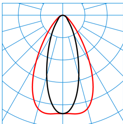
E-Line PRO 78IP50 MironaF T 270-840 ET L225 01 ESG Blank (LEO2) TX719895
