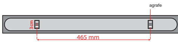
Dos du boîtier
