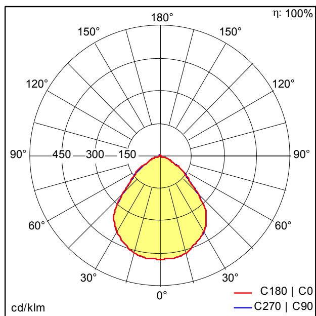
D42069AA_LF3_A_5000-940_Q_LDE_SR.Idt
