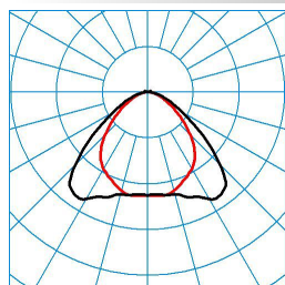
E-Line LVW160 840 L225 1 50
