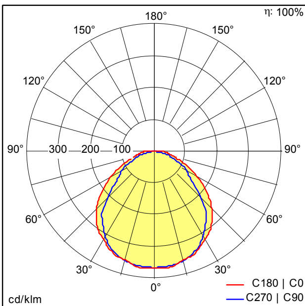
D37822AA_MLEVO_AL_LED3600-927-65_L_LDO_complete.ltd
