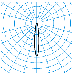
E-Line 7751 B.VEO RFS-SP-c 05 40-EW J10 ET L37 01 ■ C0 - C180 TX095684 DIN 5040: A80 UTE: 0,81 A CEN Flux Code: 100 100 100 100 81
