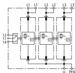
Schéma de principe du circuit DV M TNC 255 FM
