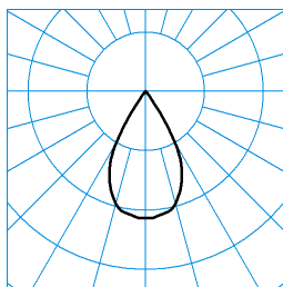
E-Line 7751 B.VEO RFS-VFL-c 05 40-BVC J07 ET L37 03 ■ C0 - C180 TX095837
