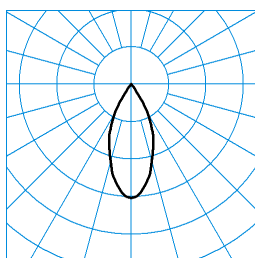
E-Line 7751 B.VEO RFS-WFL-c 05 40-BVC J07 ET L37 03 ■ C0 - C180 TX095235
