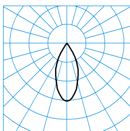
E-Line 7751 B.VEO RFS-WFL 05 40-BVC J07 ET L37 03 ■ C0 - C180 TX095893
