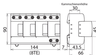
Dimensions DV M TT 255
