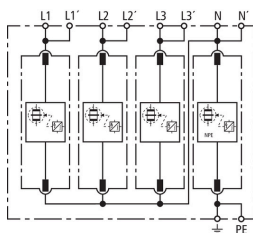
Schéma de principe du circuit DV M TT 255
