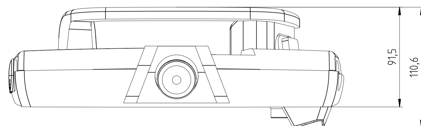
Oben / Top
