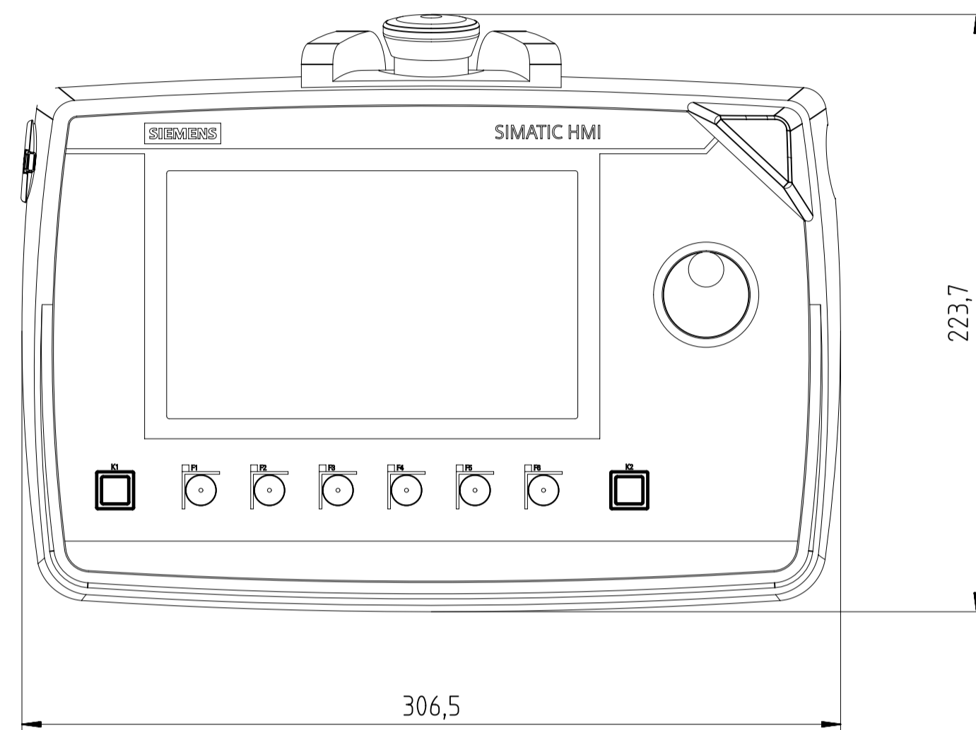
Vorne / Front
