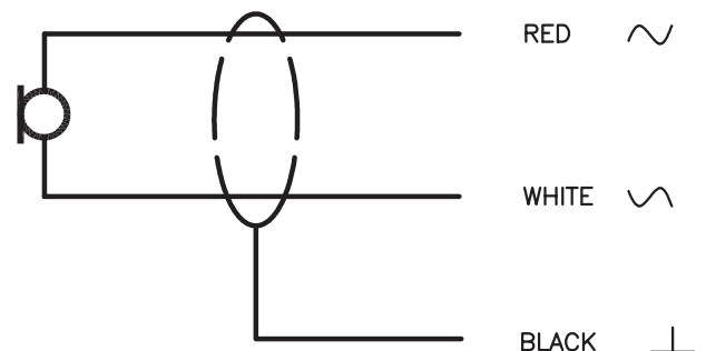
Diagramme électrique
