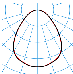
E-Line PRO 78IP50 MironaF B 200-840 ET L150 01 ESG Blank (LEO2) TX720018
