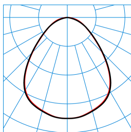
E-Line PRO 78IP50 MironaF B 200-840 ET L150 01 ESG 01 (LEO2) TX720044
