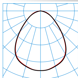
E-Line PRO 78IP50 MironaF B 200-840 ET L150 01 ESG 01 (LEO1) TX720003
