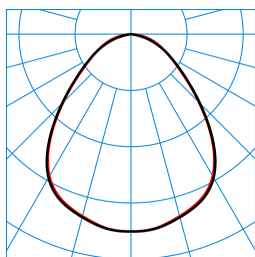
E-Line PRO 78IP50 MironaF B 200-840 ET L150 01 ESG 01 IP50 (LEO1) TX820839
