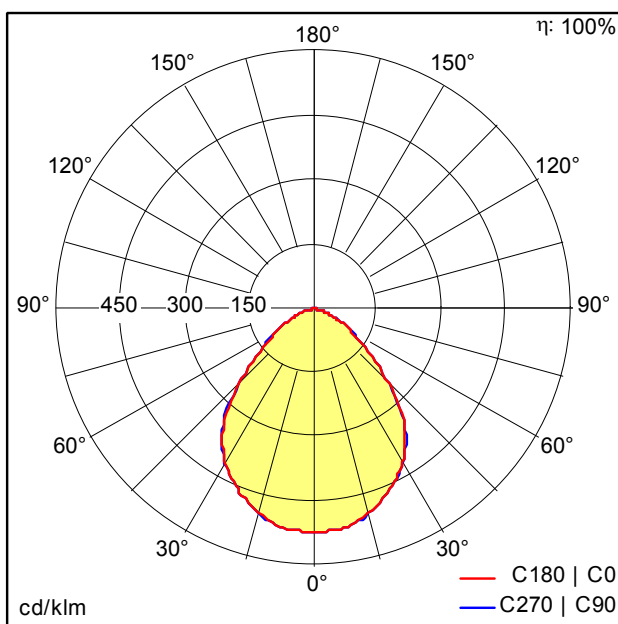
D46069_LF3_E_1600-840_M600M_EVG.Idt
