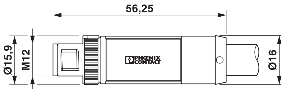
Dessin coté
